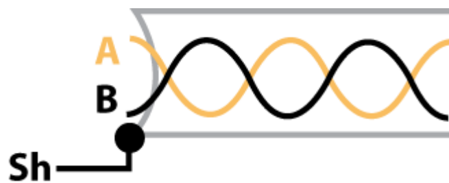
Рис. 3.12. Экранирование (интерфейс RS485)
