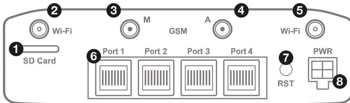
Рис. 2. Вид сзади
