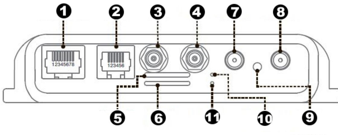
Рис. 1. Вид спереди (RL01w, RU01w)
