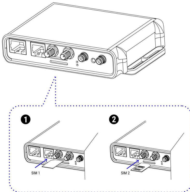
Рис. 6. Установка SIM-карт
