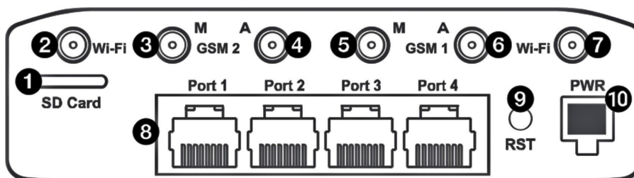
Рис. 3. Вид сзади
