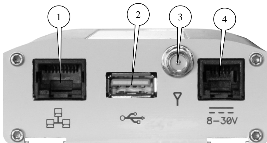
Рис.2.5.2 Вид сзади.
