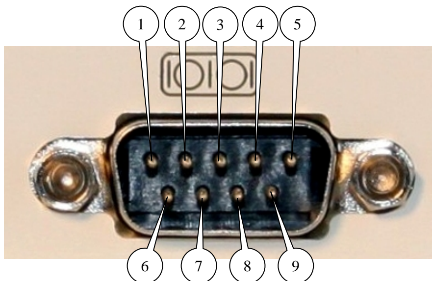
Рис.2.6.1 Разъём DB9
