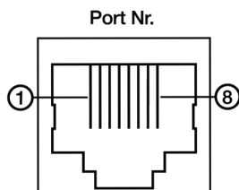
Рис. 6. Ethernet-разъем
