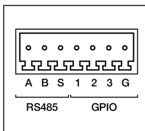
Рис. 7. Интерфейсный разъём
