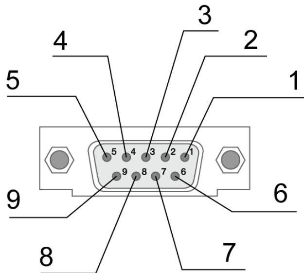
Рис. 2.3. Интерфейсный разъём
