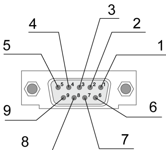
Рис. 2.5.1. Интерфейсный разъем
