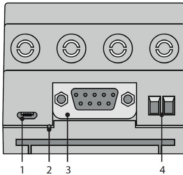
Рис. 4. Вид спереди
