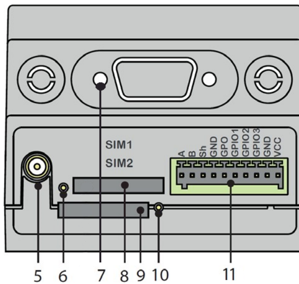
Рис. 5. Вид сзади
