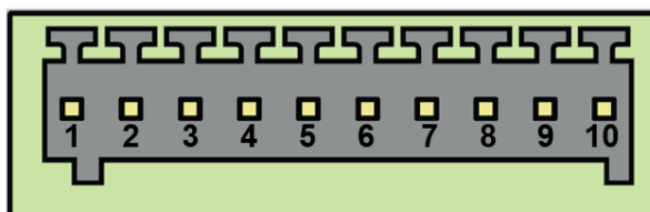
Рис. 10. Разрывной коннектор
