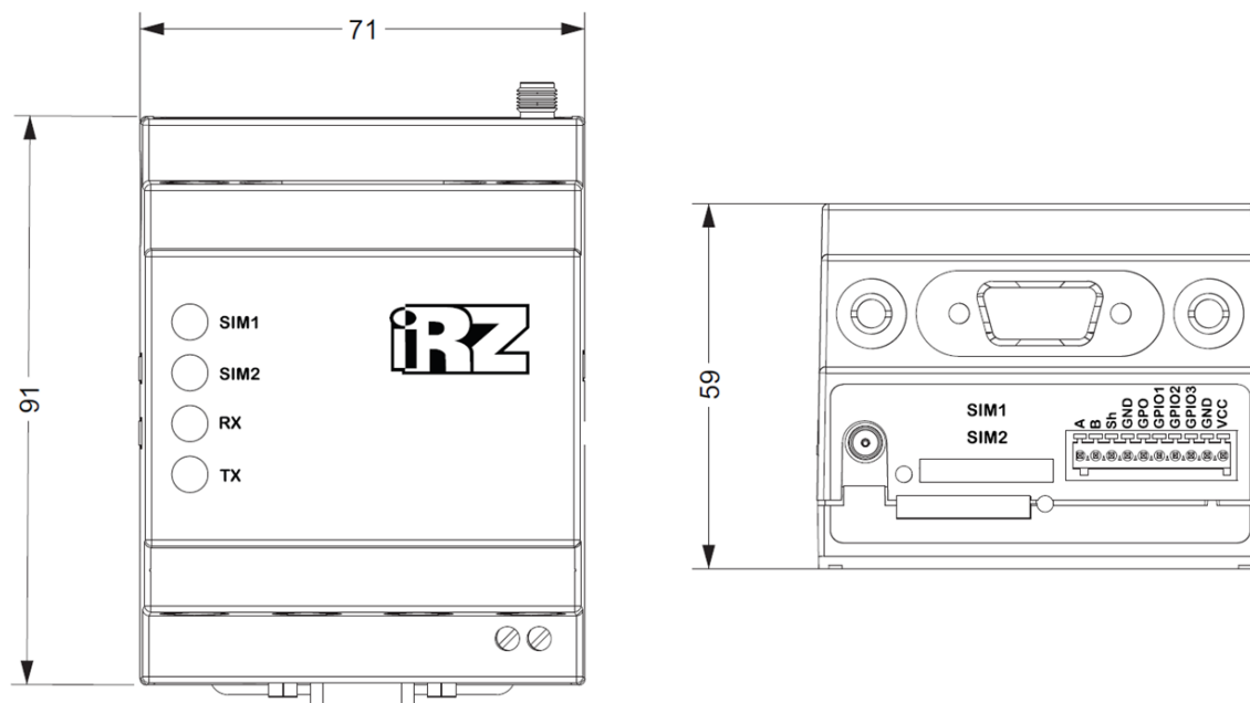
Рис. 12. Габаритные размеры модема ATM – чертёж
