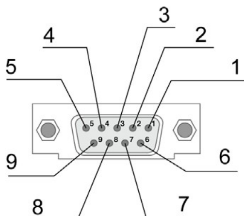
Рис. 8. Разъём DB9-F
