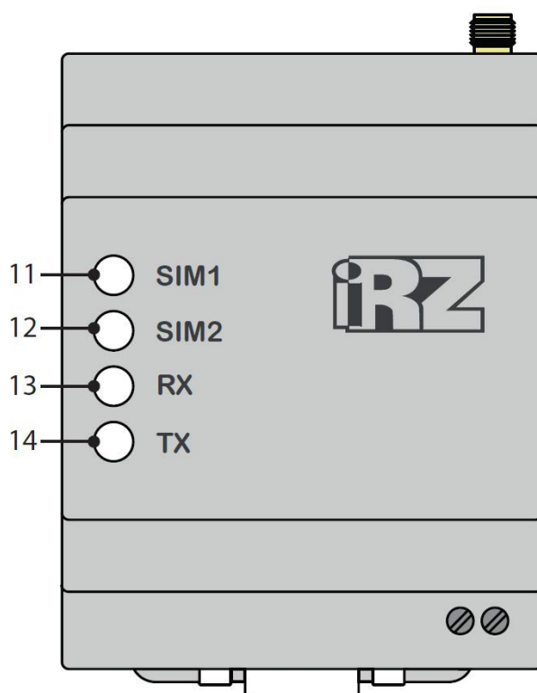
Рис. 6. Вид сверху
