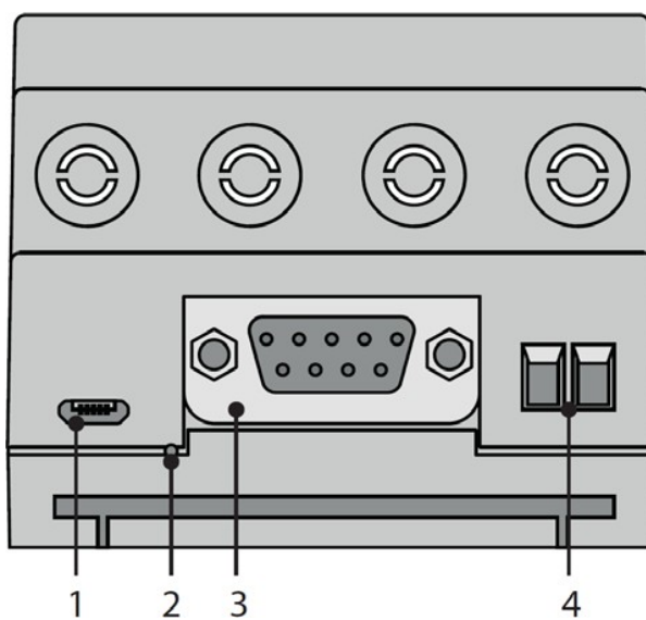
Рис. 4. Вид спереди
