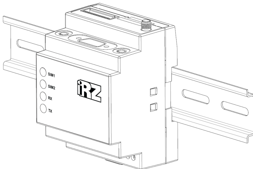
Рис. 11. Монтаж устройства – установка модема ATM на DIN-рейку
