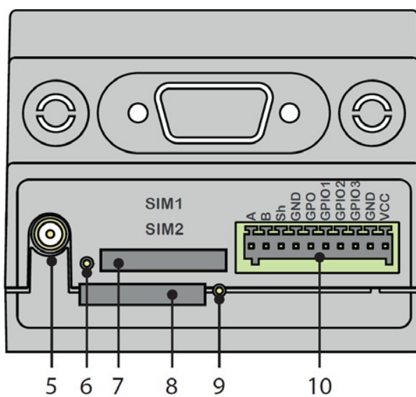
Рис. 5. Вид сзади
