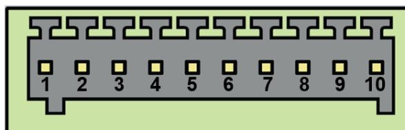
Рис. 10. Разрывной коннектор
